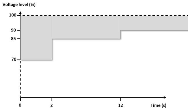
Figuur 1: Toegelaten spanningsafwijking van het spanningsniveau dat in het Aansluitingscontract van het betrokken Aansluitingspunt van de Hoofdgenerator van een Black Start PG wordt aangegeven, na de onmiddellijke overname van een afname van ten minste 10 MW.
