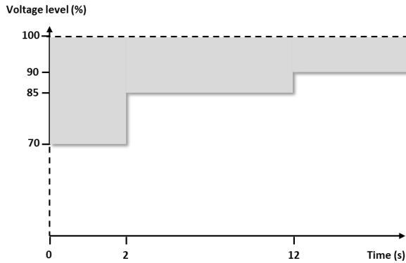
Figure 1 : Écart de tension autorisé, du niveau de tension indiqué dans le Contrat de Raccordement du P oint de R accordement en question du G énérateur P incipal d'un GF Black Start, après l'acceptation instantanée d'un prélèvement d'au moins 10 MW.
