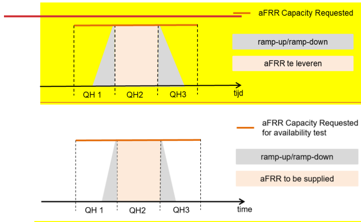
Figuur 10 - aFRR-beschikbaarheidstest
