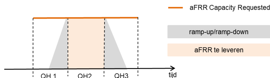
Figuur 10 - aFRR-beschikbaarheidstest
