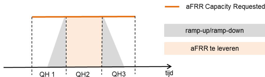
Figuur 10 - aFRR-beschikbaarheidstest
