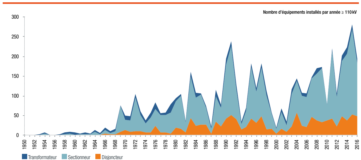
Figure 1.3 : Répartition des années de construction des principaux équipements en haute tension
