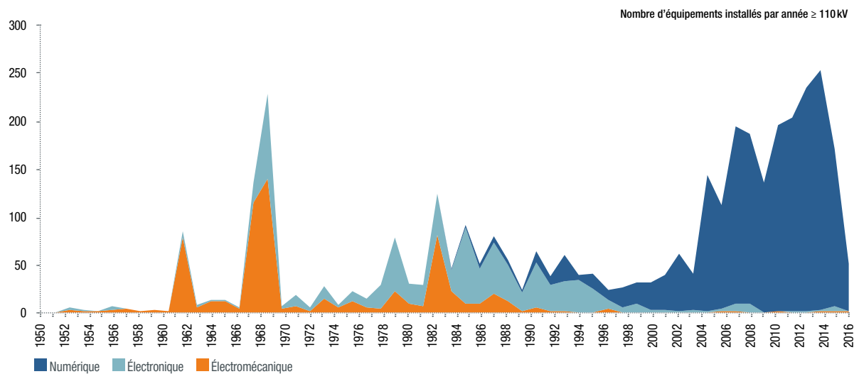
Figure 1.6: Répartition des années de construction des équipements de protection
