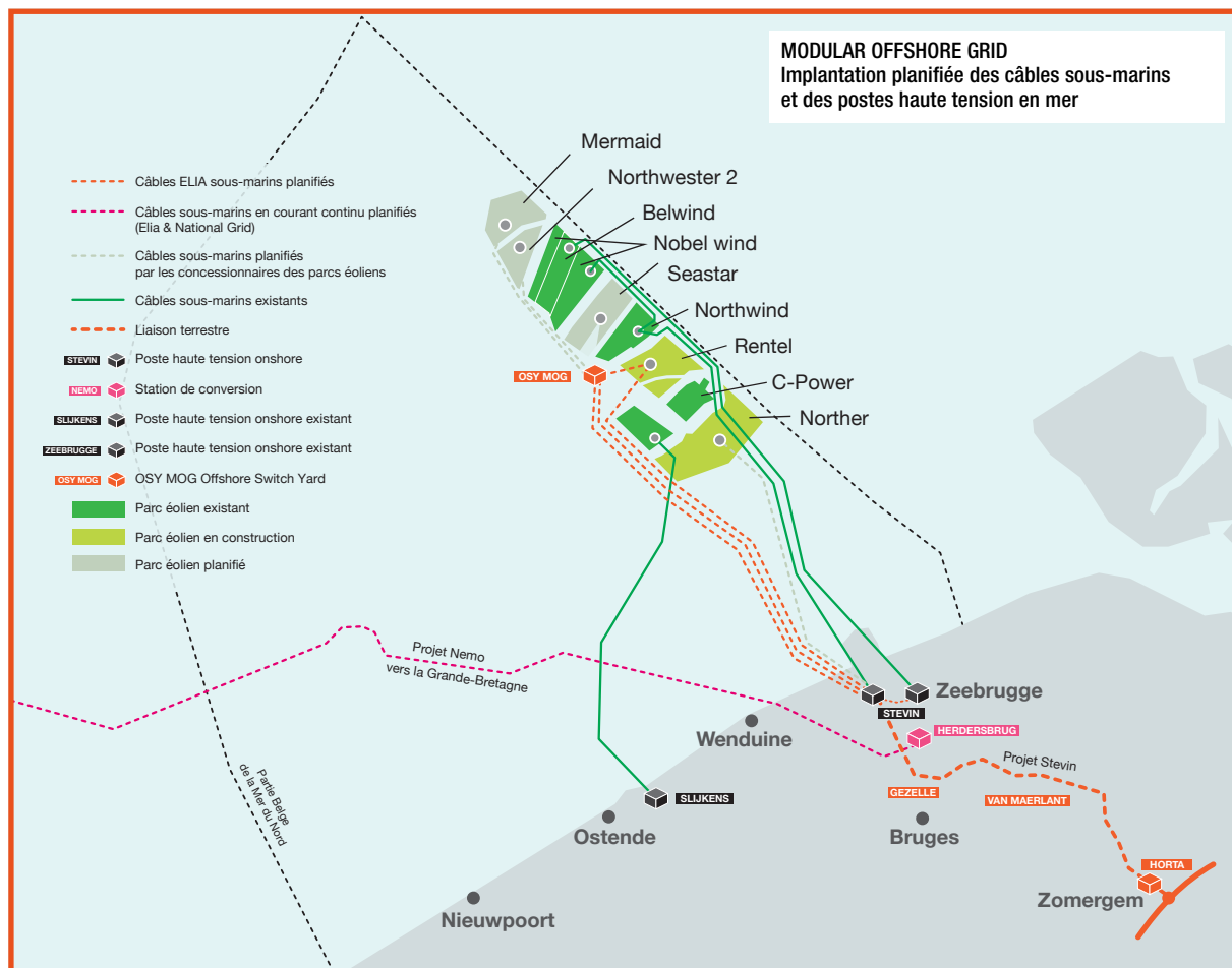
Figure 4.5 : « Prise en mer » ou « Modular Offshore Grid (MOG) »
