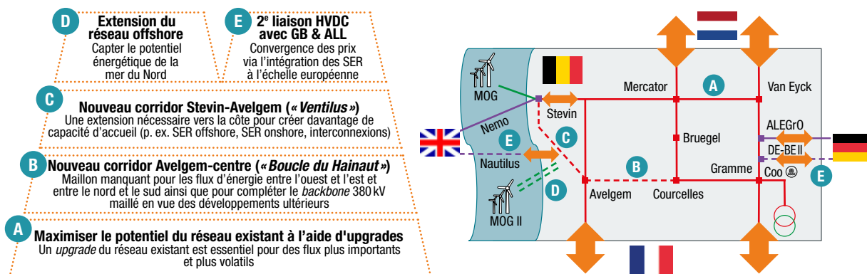
Figure 3.12 : Développement modulaire du réseau 380 kV
