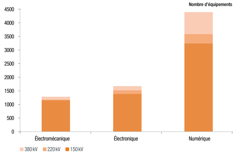
Figure 1.5: Répartition des équipements de protection en fonction de la technologie et du niveau de tension
