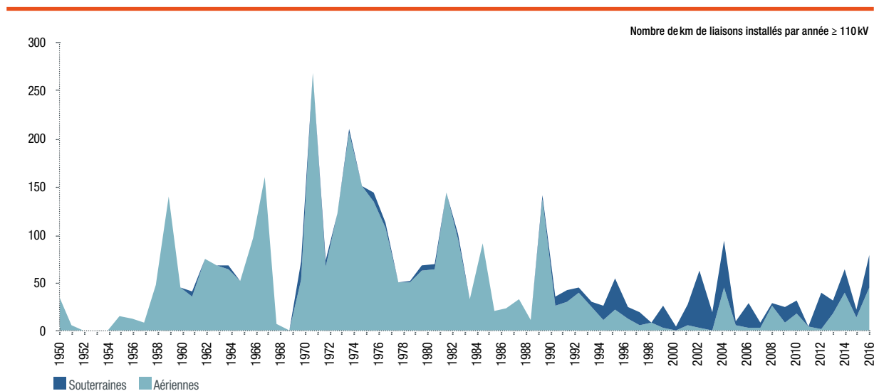
Figure 1.4 : Répartition des années de construction des liaisons
