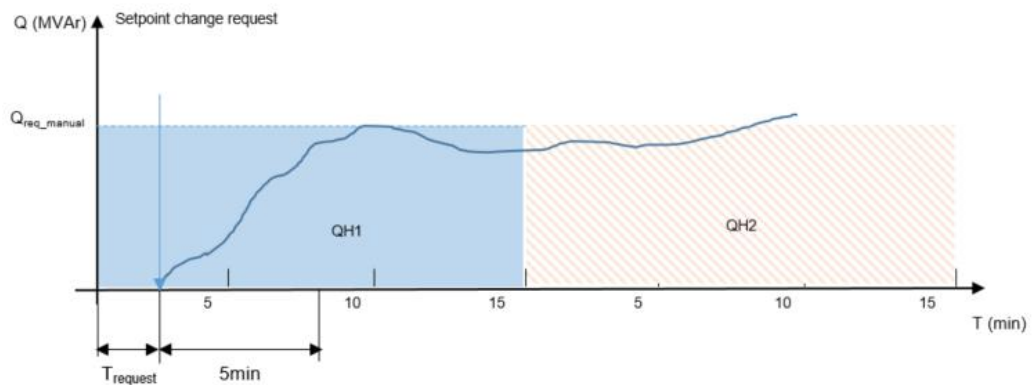
Figuur 2: Voorbeeld van de berekening van Q_{reqrem,q} voor een kwartier waarin een aanvraag tot wijziging van de Referentiewaarde is doorgegeven voordat binnen dat kwartier 10 minuten verstreken zijn
