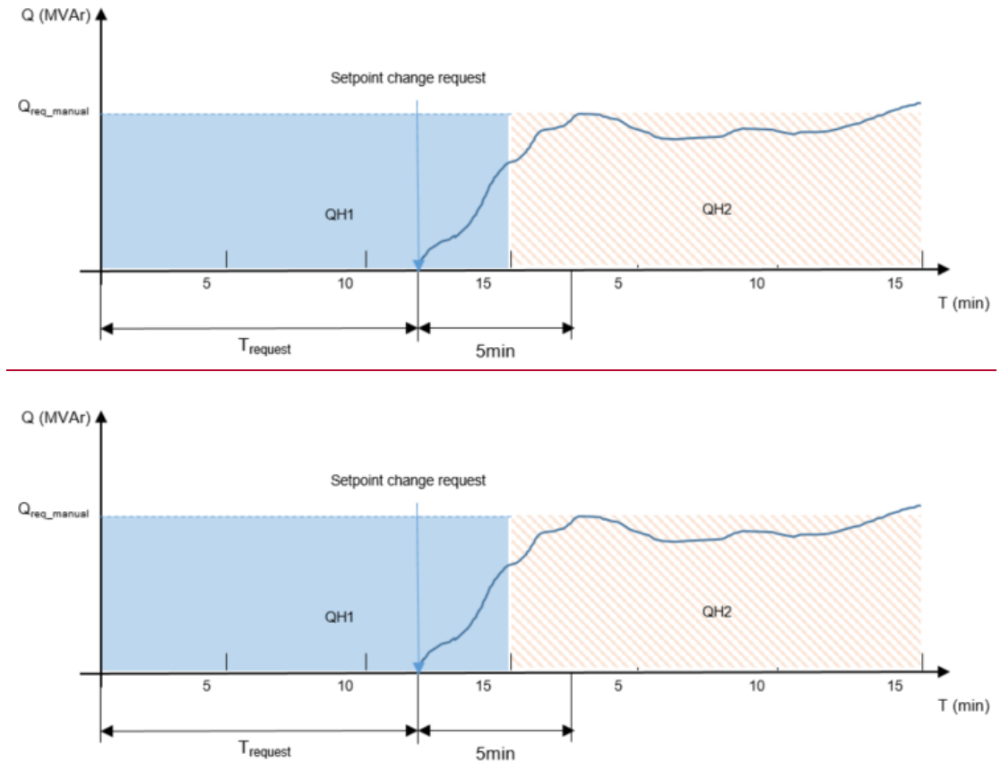
Figuur 3: Voorbeeld van de berekening van Q_{req\_rem} voor 2 kwartieren waarin een aanvraag tot wijziging van de Referentiewaarde is doorgegeven nadat binnen het eerste kwartier 10 minuten verstreken zijn
