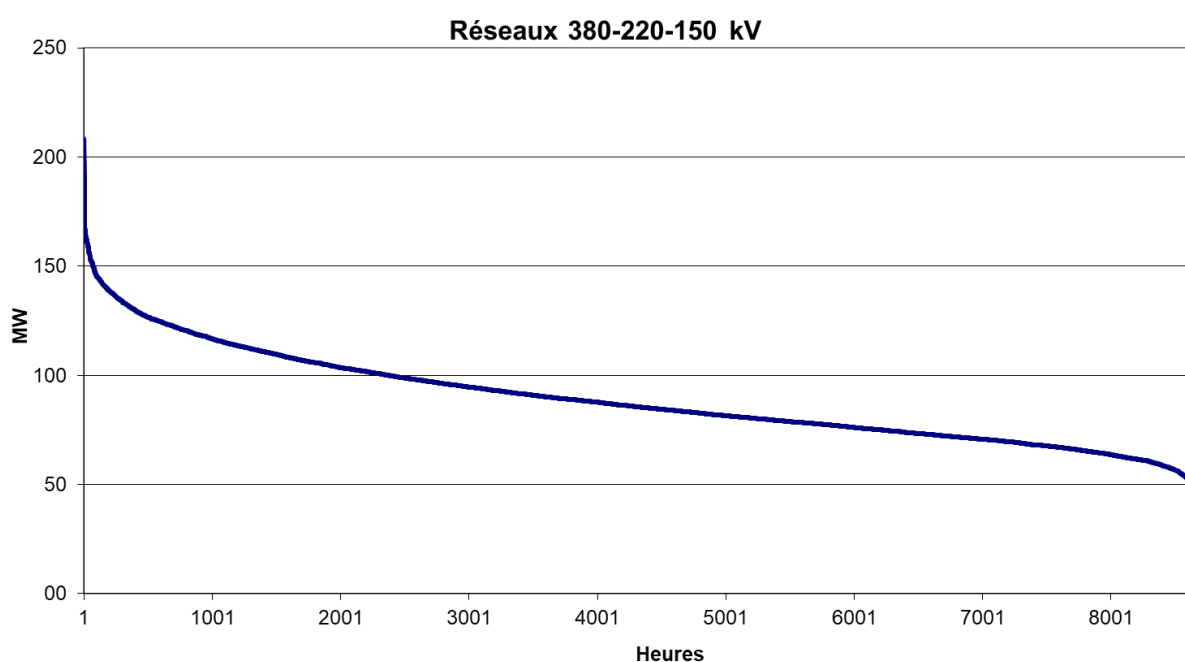
Courbe monotone des pertes 2019
