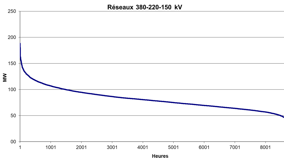
Courbe monotone des pertes 2020
