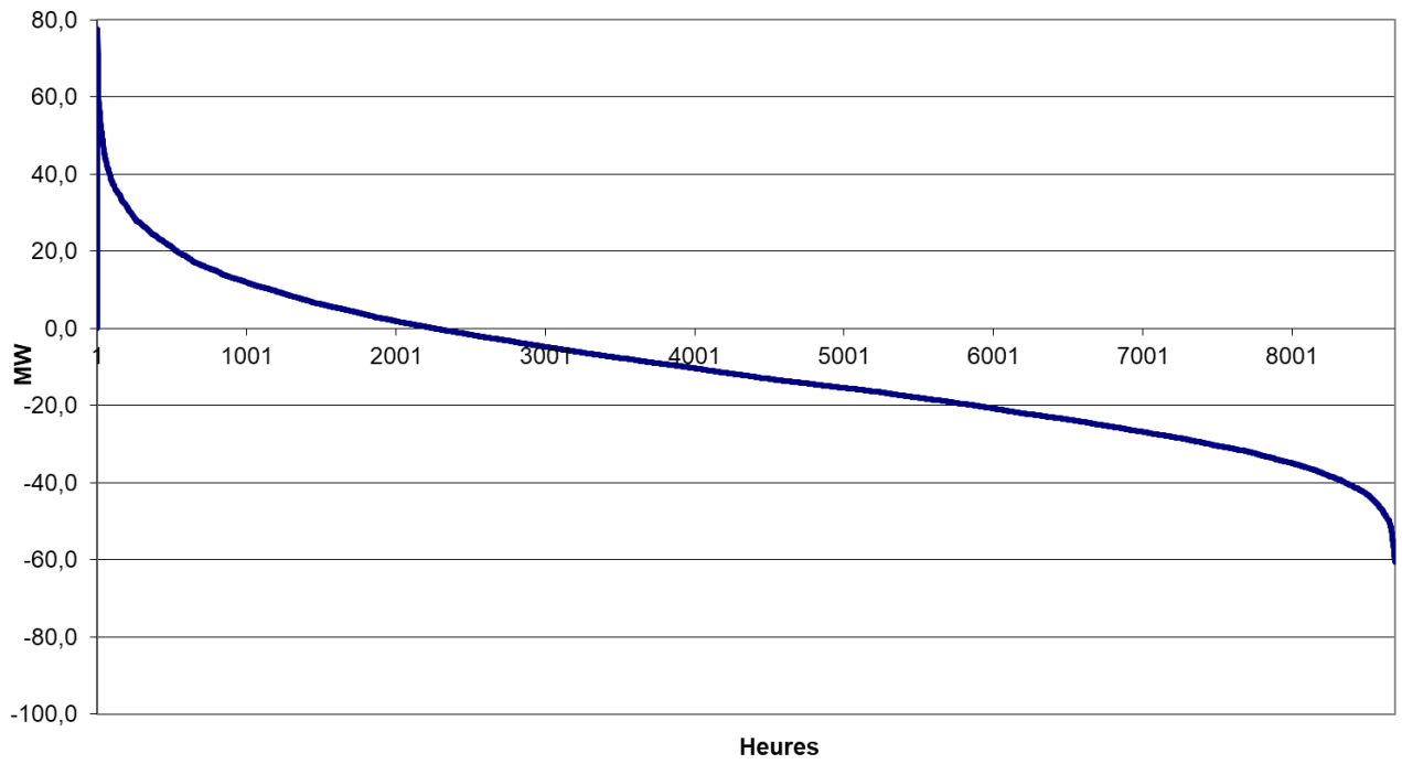
Courbe monotone du déficit de compensation 2020
