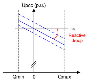
Upccgeeft de spanning weer op het aansluitingspunt
