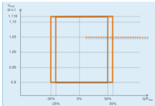
U-Q/PD-profiel voor SPM van het type C & D: vereisten met betrekking tot het reactief vermogen voor verschillende spanningniveaus vanaf 1pu (gestippeld voor nominale spanningen boven 300kV).
